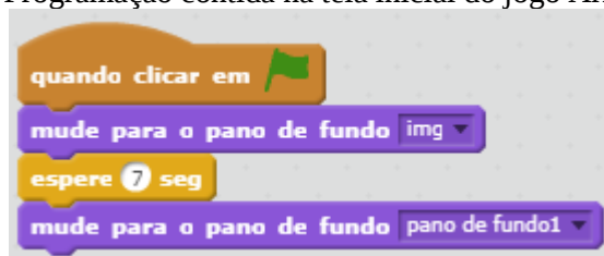
Figura 18 - Programação contida na tela inicial do jogo Arruma Sílabas
