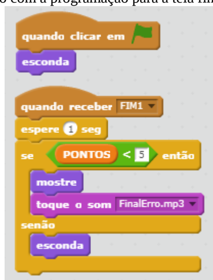
Figura 16 - Bloco com a programação para a tela final de erro do jogo
