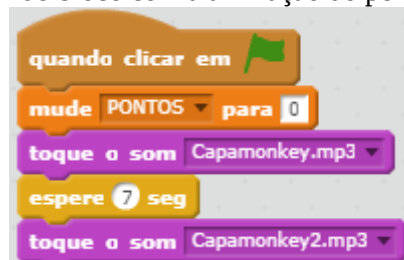
Figura 22 - Segundo bloco com a animação do personagem Monkey
