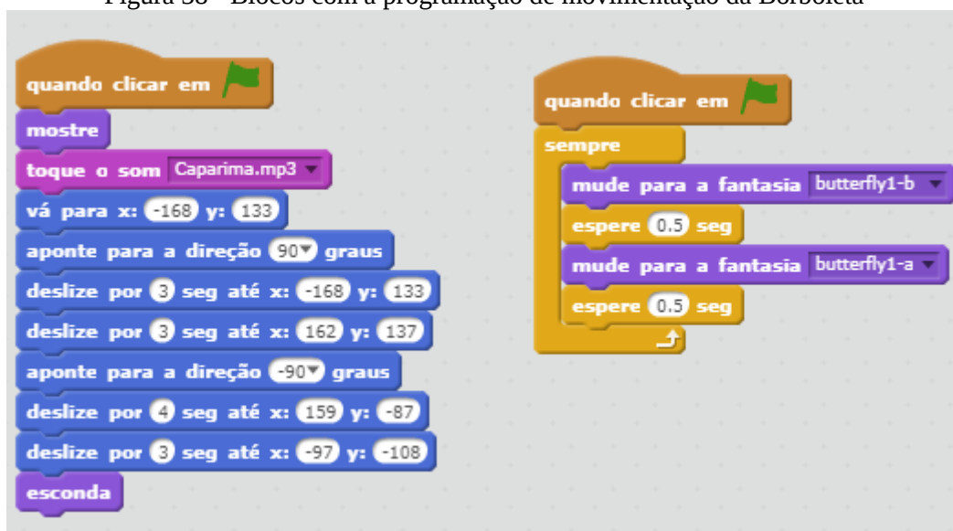
Figura 38 - Blocos com a programação de movimentação da Borboleta
