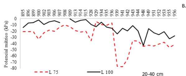
Figura 1. Os valores médios de potencial matricial (kPa) na camada de 0-20 cm (A) e de 20-40 cm do solo (B), cultivado com mamoeiro, em função dos dias após transplante e das lâminas de irrigação aplicadas (75% e 100% da ETc), em Juazeiro-BA.2019.
