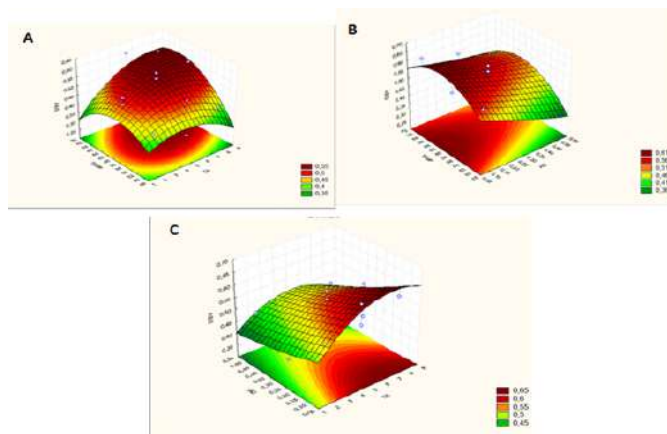
Figura 1. Superfície de resposta para rendimento de sólidos solúveis em função dos fatores (A) proporção tempo de agitação e temperatura, (B) temperatura e acidificação, (C) acidificação e tempo de agitação.
