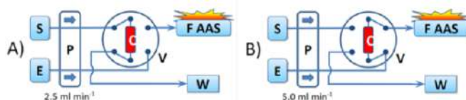
Figura 1: Diagrama esquemático do sistema de extração e pré-concentração em linha desenvolvido para determinação de Pb por F AAS: A = etapa de amostragem; B = etapa de eluição; C = mini-coluna empacotada com nanopartículas de CoFe 2 O 4 revestidas com TAR; E = solução do eluente (HCl 0,10 mol L -1 ). S = amostra ou solução padrão; P = bomba peristáltica; V = válvula de seis vias; W = descarte.
