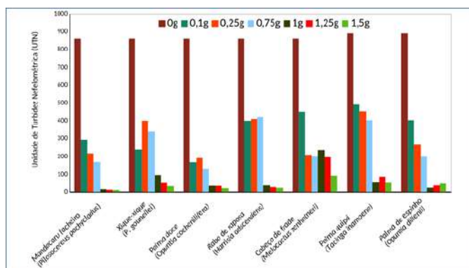
Figura 2. Redução da turbidez da água bruta de barragem após tratamento com diferentes espécies de cactáceas da caatinga, com concentração variando entre 0 (sem tratamento) e 1,5% (P/V).
