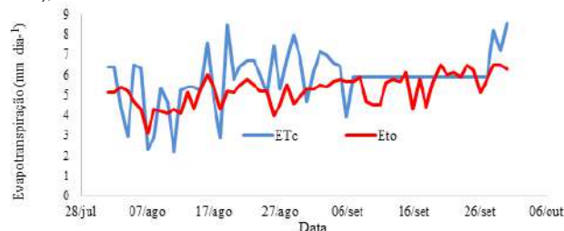
Figura 2. Variação da Evapotranspiração da cultura e referência (A), em função das datas, em Juazeiro-BA.2019.
