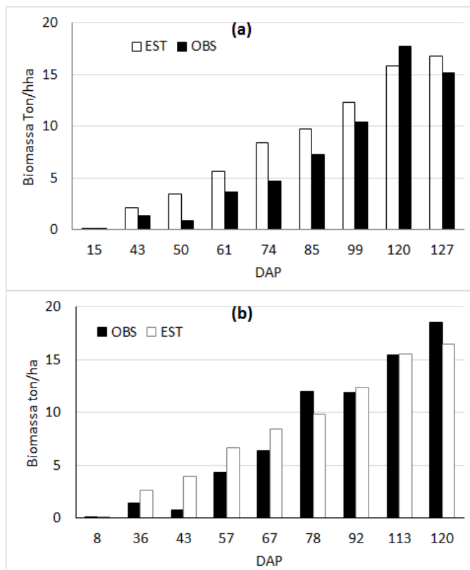
Figura 1. Evolução da Produção de Biomassa observada e estimada pelo modelo AquaCrop, em função do DAP, para a cultura da soja, cultivar M8349: a) Pivot 4 e b) Pivot 16.
