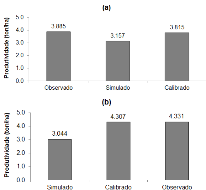
Figura 1. Produtividade observada, simulada e calibrada pelo modelo AquaCrop para a cultura da soja, cultivar M8349: a) Pivot 4 e b) Pivot 16.
