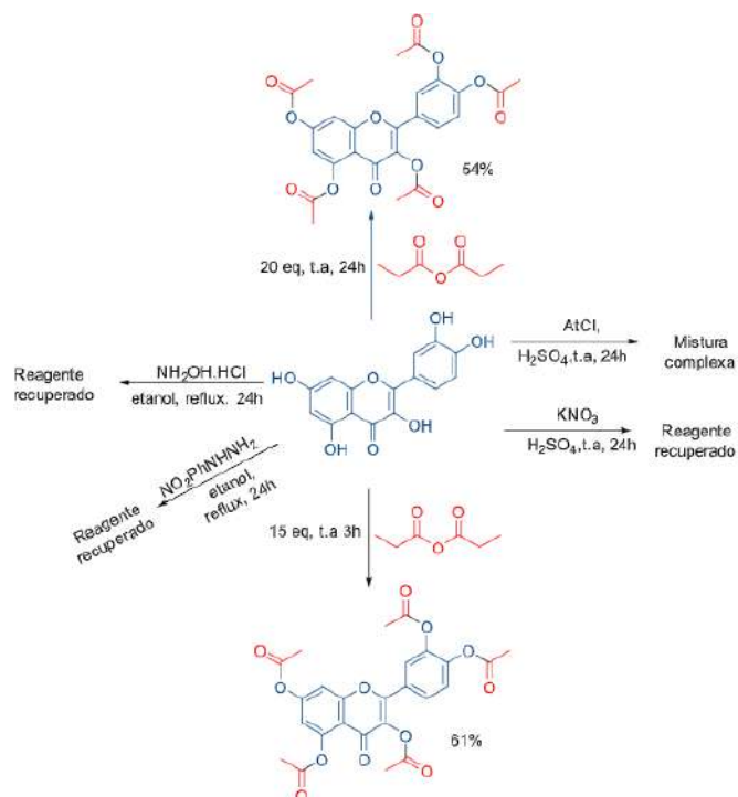
Figura 2. Reações de modificação da quercetina.
