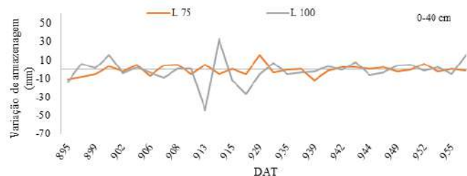
Figura 3. Variação do armazenamento de água (mm) na camada de 0-40 cm, em função dos dias após transplante e das lâminas de irrigação aplicadas (75% e 100% da ETc) para o mamoeiro, em Juazeiro-BA.2019.
