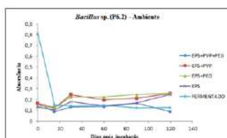
Figura 1. Expressão linearizada das concentrações de células da estirpe Bacillus sp. (P6.2) nas cinco diferentes formulações a base de EPS e aditivadas com PVP e PEG em função dos dias de incubação, mantidos em temperatura ambiente.
