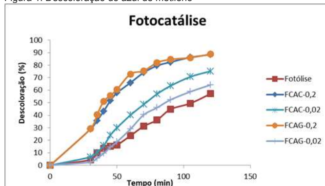
Figura 1. Descoloração do azul de metileno
