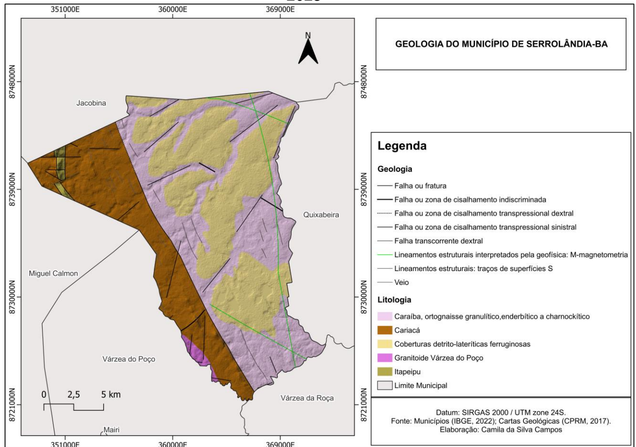
Figura 16 – Mapa de Unidades Litoestratigráficas do município de Serrolândia- BA, 2023
