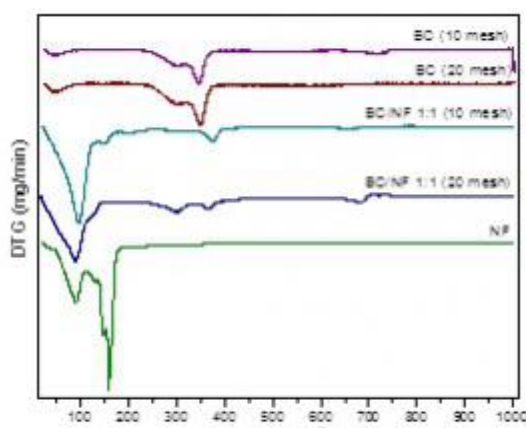
Figura 1. Curvas DTG
