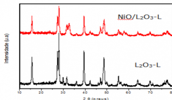
Figura 2 - Perfis de DRX dos sólidos.
