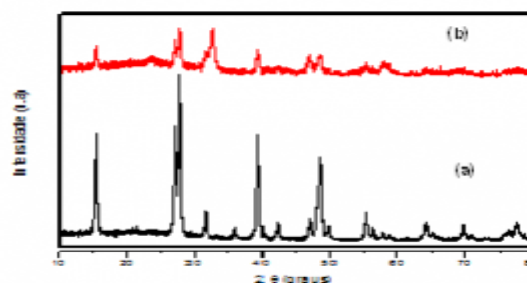
Figura 2. Perfis de DRX das amostras obtidas.
