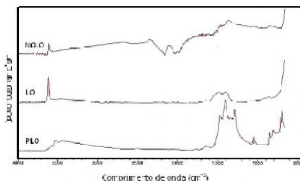
Figura 1. Espectro de FTIR das amostras obtidas.
