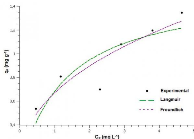
Figura 2. Isoterma de adsorção do azul de metileno sobre a amostra BC/NF 1:1
