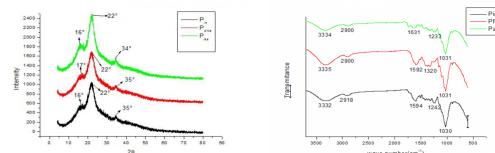
Figura 1. DRX e FTIR das amostras Pin, PbNa, e Pas
