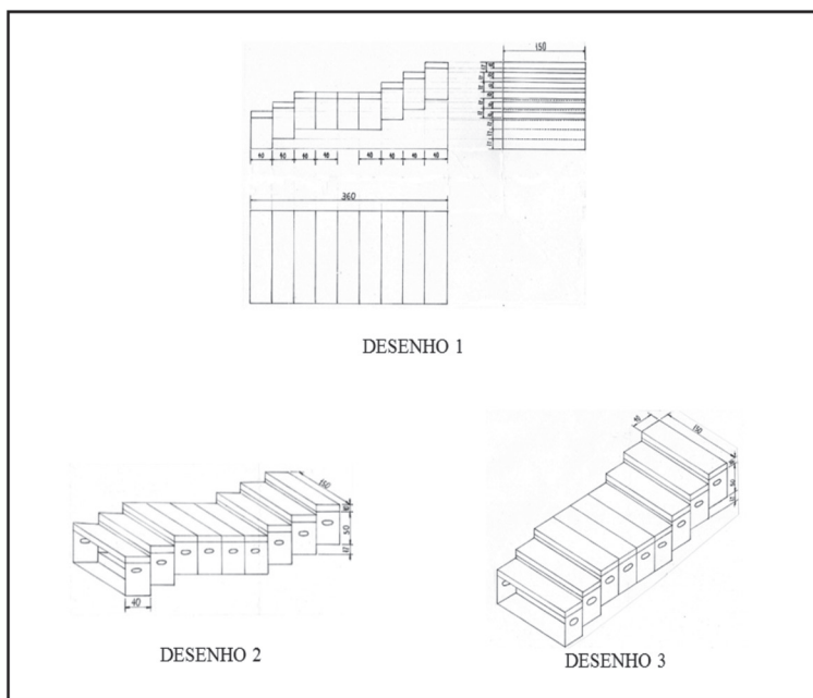
Figura 4 – Desenho Técnico do elemento representado pela equipe
